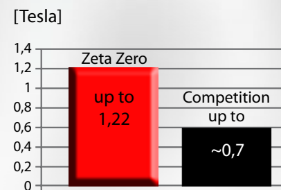
Внутренняя индукция и напряженность магнитного поля Gap Flux & Force [Tesla]
